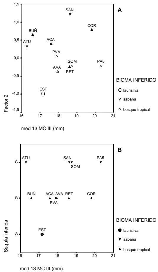
Fig. 6.- a) Valor medio de la variable 13MCIII ( sensu EISENMANN et al. , 1988) en relación con el valor del componente 2 del ACP en poblaciones de Anchitherium ibéricas (y Sansan). b) Valor medio de la variable 13MCIII ( sensu EISENMANN et al. , 1988) en relación con la duración de la sequía, inferida a partir del análisis discriminante, en poblaciones de Anchitherium españolas (y Sansan). Siglas como en Tablas 2 y 10. Leyenda como en la Fig. 5.
