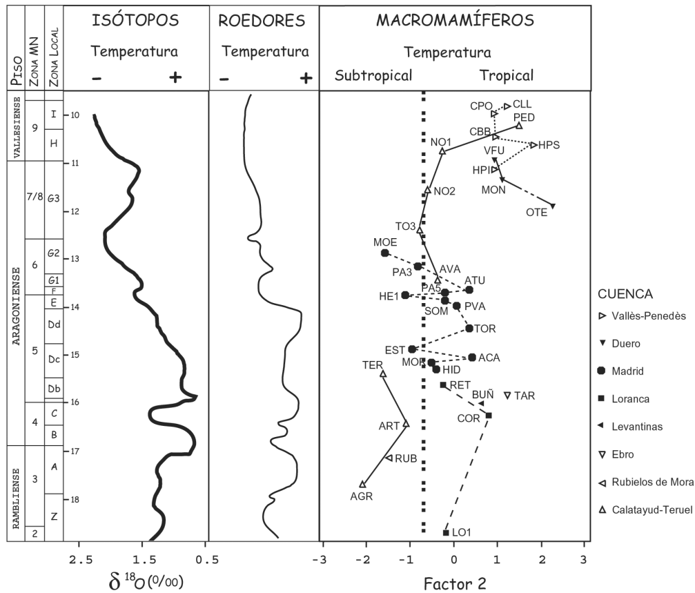
Fig. 4.- Variación temporal del valor obtenido en el segundo componente del ACP en los yacimientos estudiados separando las diferentes cuencas españolas. Se compara con las variaciones de temperatura propuestas a partir del análisis de las faunas de roedores realizado por VAN DER MEULEN & DAAMS (1992) y ALCALÁ et al. (2000) y con la curva isotópica del O18 para el lapso temporal estudiado (FLOWER, 1999). La ubicación temporal de los yacimientos es aproximada.
