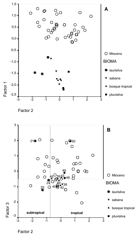
Fig. 1.- a) Distribución de las faunas actuales y fósiles en función de los componentes 1 y 2 del ACP. b) Distribución de las faunas actuales y fósiles en función de los componentes 2 y 3 del ACP. Datos estadísticos en la Tabla 5. Números como en la Tabla 3.
