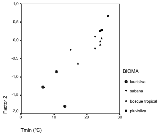
Fig. 2.- Temperatura media del mes más frío (Tmin) en localidades actuales en relación con el valor del componente 2 del ACP. Fig. 2.- Coldest month mean temperature (Tmin) in recent localities plotted to component 2 value of PCA.
