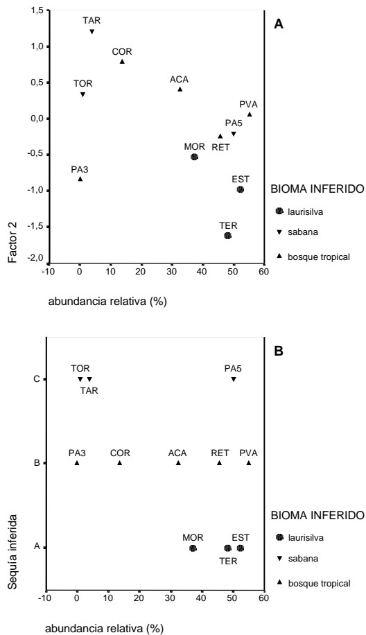
Fig. 8.- a) Abundancia relativa de Anchitherium (% del total de la fauna de macromamíferos) en relación con el valor del componente 2 del ACP en yacimientos españoles del Aragoniense. b) Abundancia relativa de Anchitherium (% del total de la fauna de macromamíferos) en relación con la duración de la sequía, inferida a partir del análisis discriminante, en yacimientos españoles del Aragoniense. Los datos de abundancia relativa proceden de ALFÉREZ et al. (1982), MORALES et al. (1993) y AMEZUA et al. (2000). Siglas como en Tablas 2 y 10. Leyenda como en la Fig. 5.
