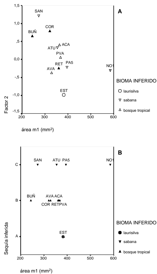
Fig. 5.- a) Área del primer molar inferior (área m1) en relación con el valor del componente 2 del ACP en poblaciones de Anchitherium españolas (y Sansan). Símbolos negros, primer clado según SÁNCHEZ et al. (1998); símbolos blancos, segundo clado; símbolos grises, A. sampelayoi (clado indeterminado). b) Área del primer molar inferior (área m1) en relación con la duración de la sequía inferida a partir del análisis discriminante en poblaciones de Anchitherium españolas (y Sansan): A, sin sequía (laurisilva); B, sequía moderada (bosque tropical); C, sequía prolongada (sabana). Siglas como en Tablas 2 y 10. Biomas inferidos como en Fig. 3. Fig. 5.- a) Lower first molar mean area (área m1) plotted to component 2 of PCA value in Spanish (and Sansan) samples of Anchitherium . Black symbols, first clade after SÁNCHEZ et al. (1998); white symbols, second clade; grey symbols, A. sampelayoi (indetermined clade). b) Lower first molar mean area (área m1) plotted to inferred dry period duration from discriminant analysis in Spanish (and Sansan) samples of Anchitherium . Sequía inferida (inferred dry period): A, no drought; B, moderate drought; C, prolonged drought. Abbreviations as in Tables 2 and 10. Inferred biomes as in Fig. 3.
