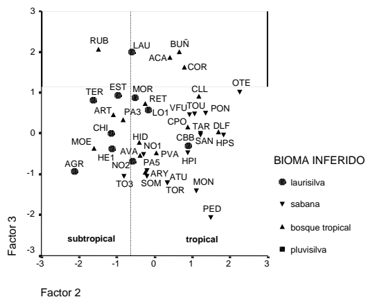
Fig. 3.- Biomas inferidos para las faunas de macromamíferos del Mioceno, distribuidas en función de los componentes 2 y 3 del ACP. Siglas como en las Tablas 2 y 10.
