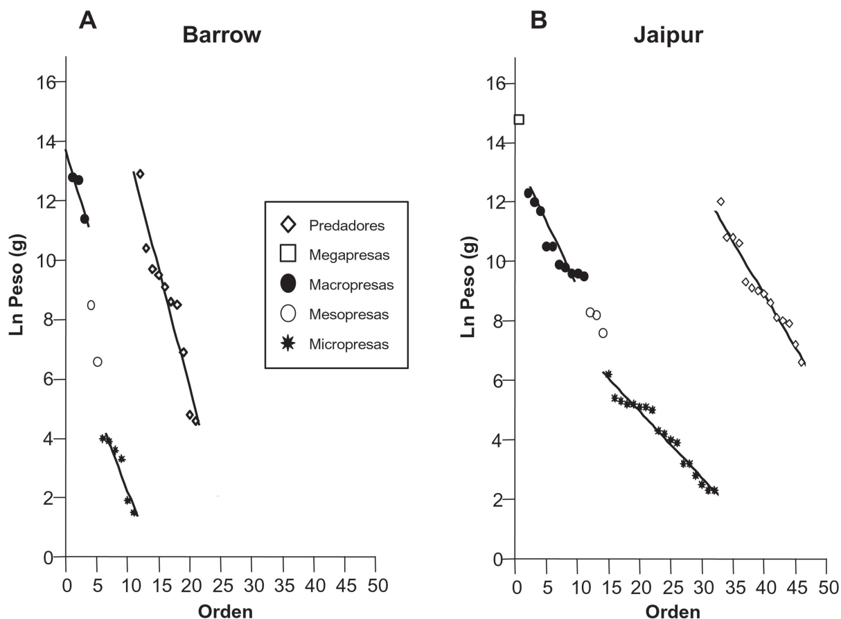
Fig. 2.— A: Cenograma de la comunidad de Barrow (Alaska). B: Cenograma de la comunidad de Jaipur (India).
