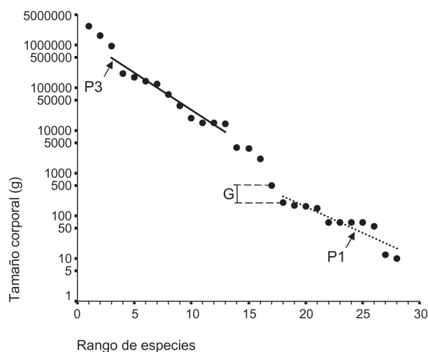
Fig. 1.—Cenograma de la fauna de mamíferos modernos de Patna, India.
