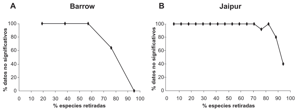
Fig. 4.—Porcentaje de pseudocomunidades que no muestran diferencias significativas frente a la comunidad original en un análisis de \chi^2 , dentro de cada categoría de porcentaje de especies eliminadas. A: Barrow. B: Jaipur.
