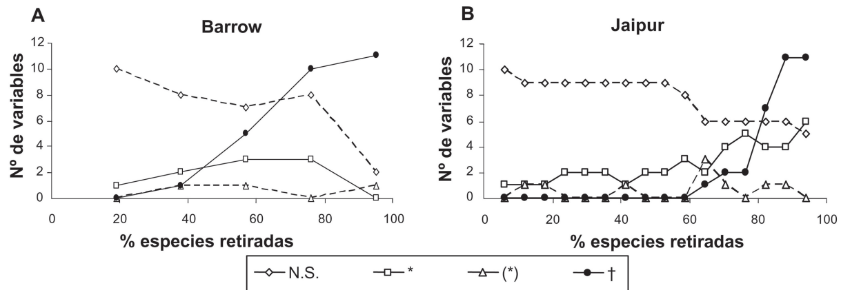
Fig. 3.—Número de variables del cenograma (tabla 1) que no muestran diferencias significativas (N.S.) entre las pseudocomunidades y la comunidad original, en un análisis de Monte Carlo, dentro de cada categoría de porcentaje de especies eliminadas. También se indican las que muestran diferencias significativas *, diferencias marginalmente significativas (*) y en las que se han perdido datos †. A: Barrow. B: Jaipur.
